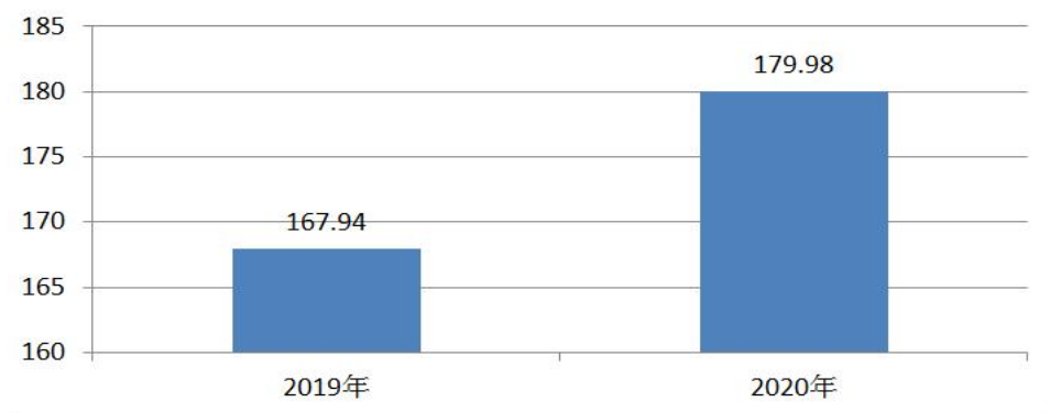
图五：2020年财政拨款支出决算变动情况（单位：万元）
